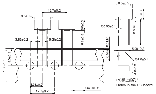
Dimensions / 尺寸图 (Unit / 单位:mm)
